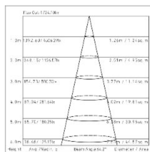
Nota: Las curvas indican el área iluminada y la iluminancia promedio según la distancia de la luminaria.
